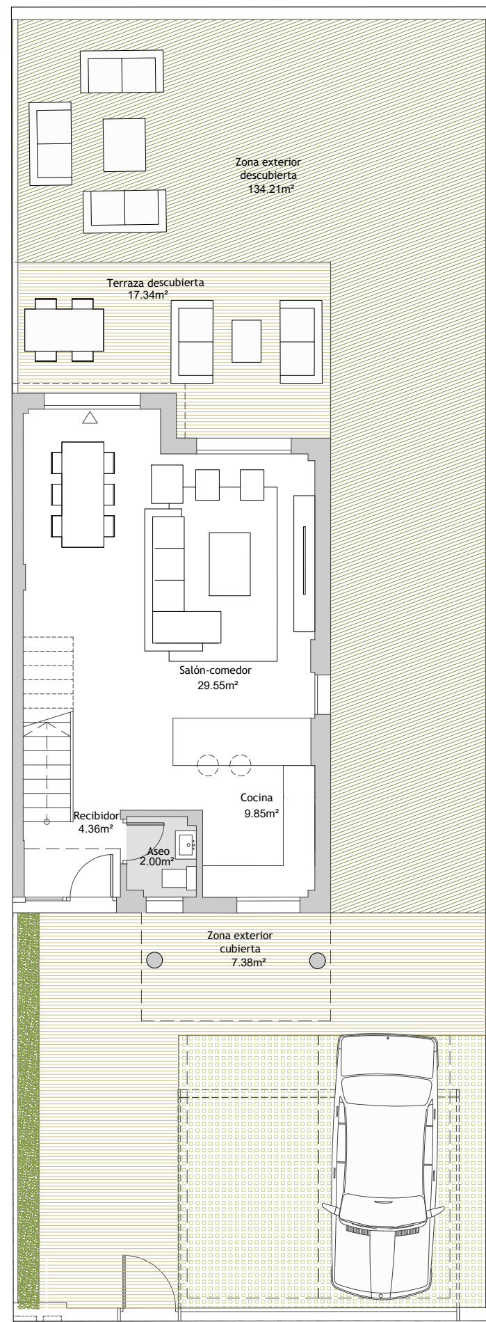
PLANTA BAJA
